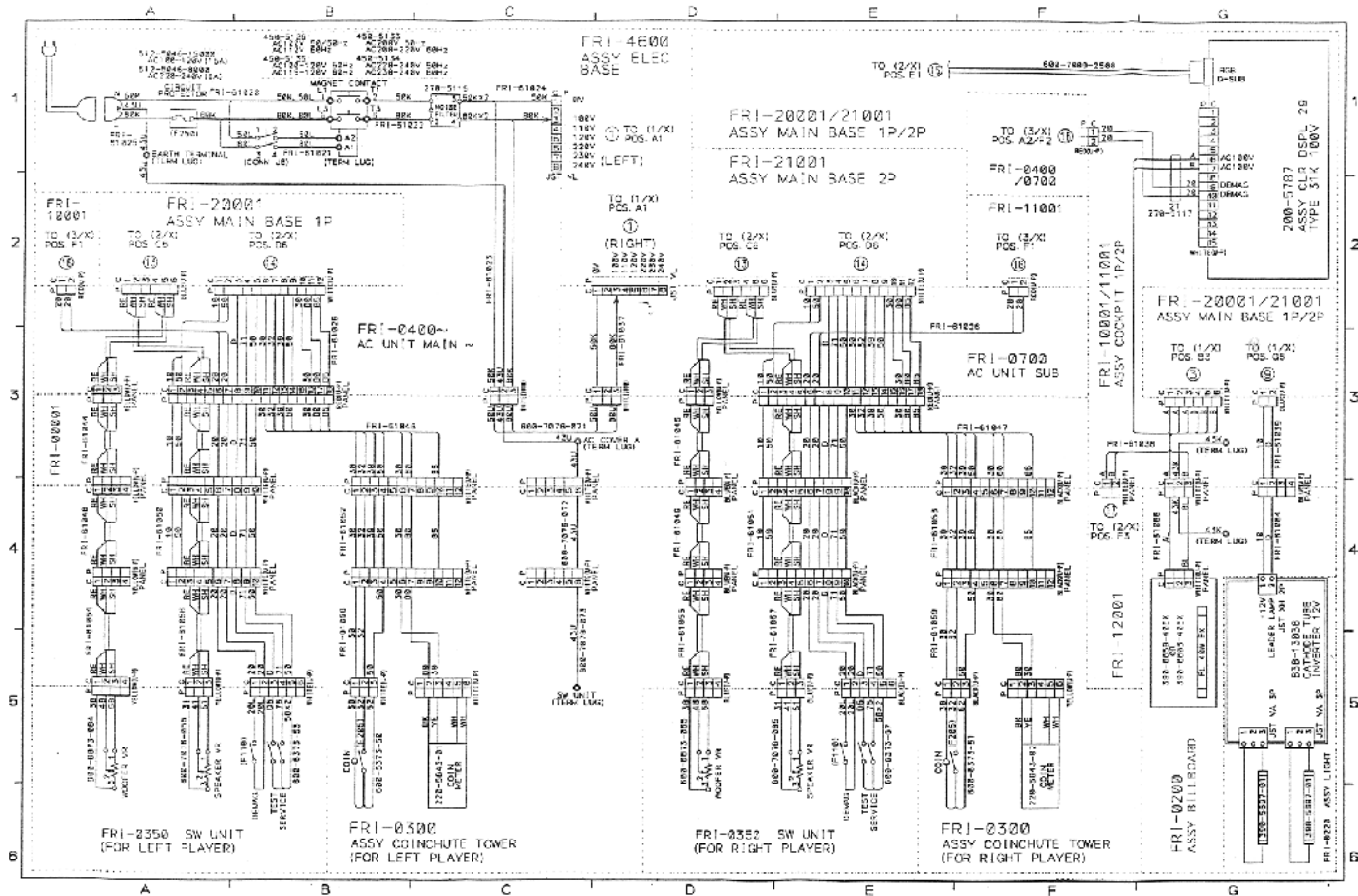
23. WIRING DIAGRAM (D-3/5)
